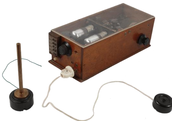
Рисунок 4. Терменвокс системы Ковальского
