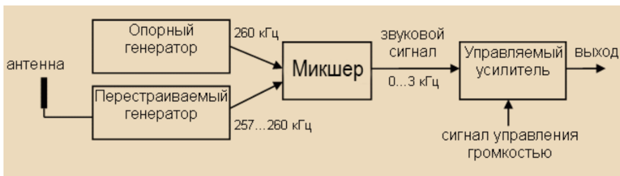
Рисунок 2. Схема устройства терменвокса
