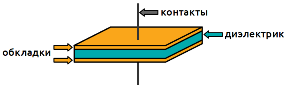
Рисунок 1. Схема устройства конденсатора
